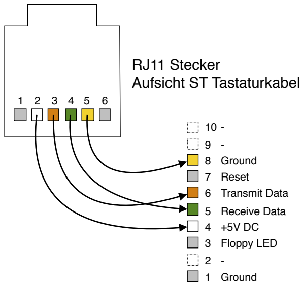
Abbildung 1: Mega ST(E)/TT Tastaturkabel
