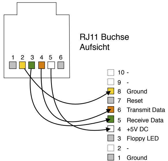
Abbildung 2: Verwendung einer RJ11 Buchse am Falcon
