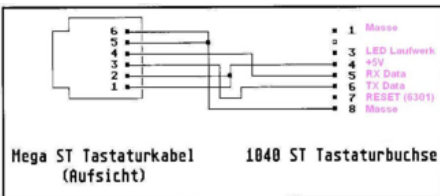
Abbildung 3: Mega ST(E)/TT Tastaturkabel an 1040 ST Tastaturbuchse
